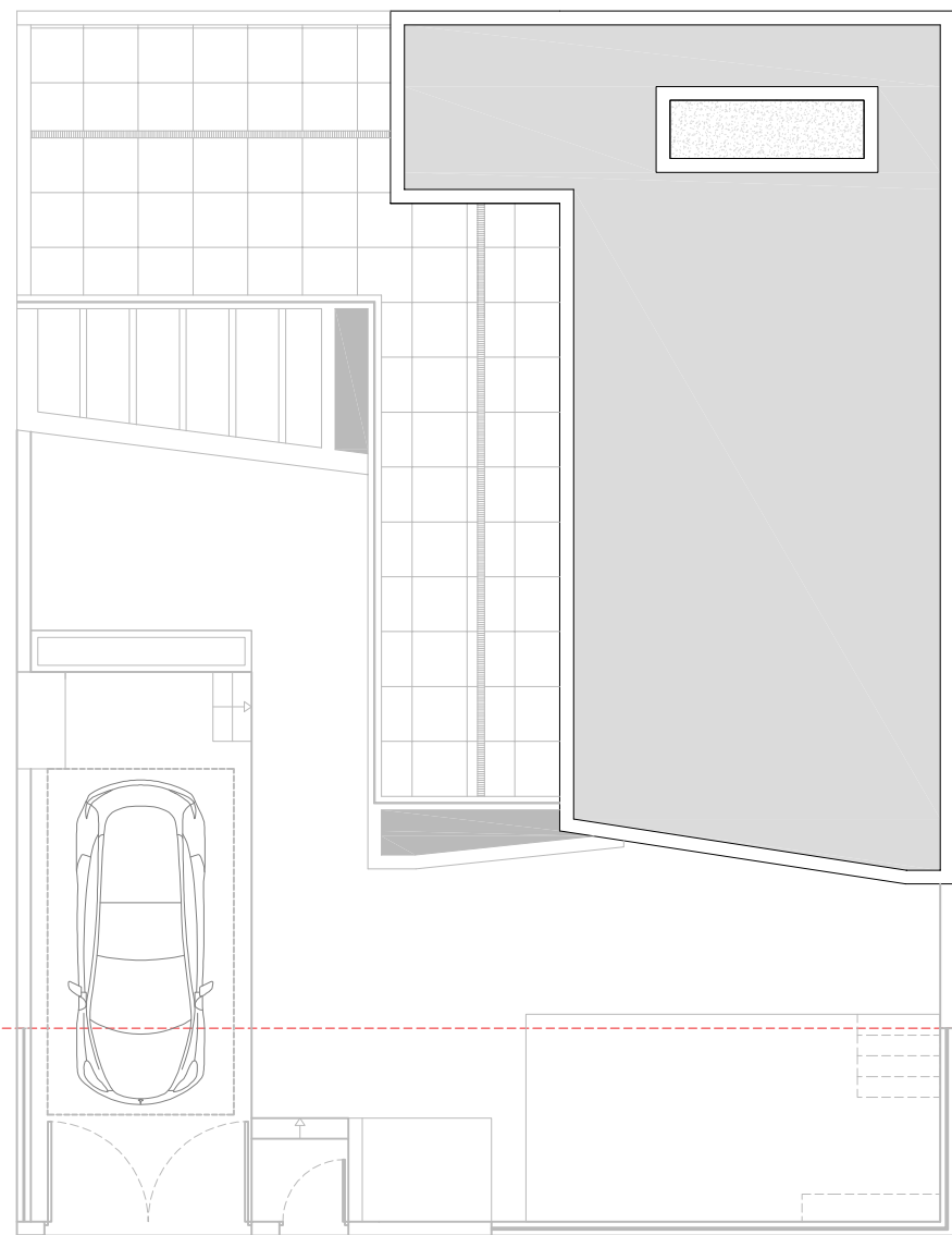
PLANTA CUBIERTA VIV 4, 5 Y 6
