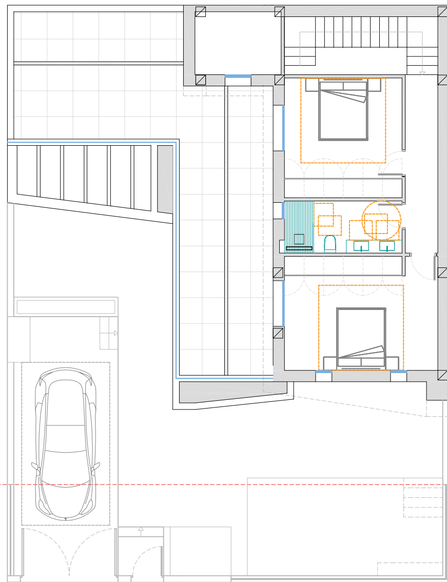
PLANTA PISO VIV 4, 5 Y 6
